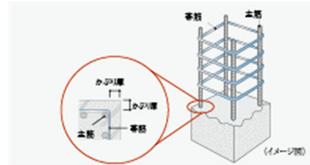
■かぶり厚測定～確保
