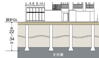
■ 基礎概念図
