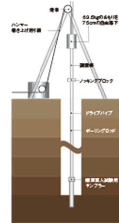
■ 貫入試験概念図
