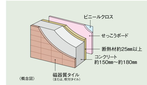
■外壁概念図
