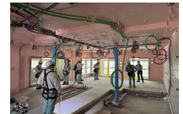
■排水堅管
