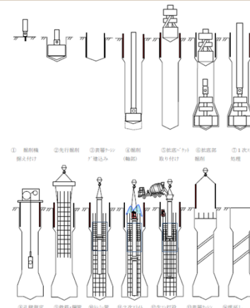
■ 杭概念図
