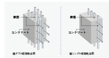
■ダブル配筋
