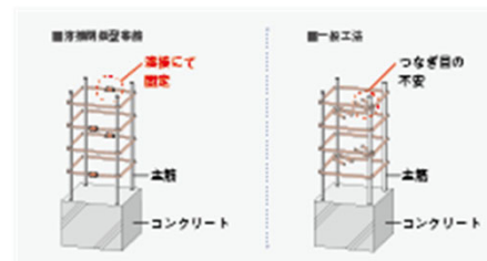
■溶接閉鎖型帯筋
